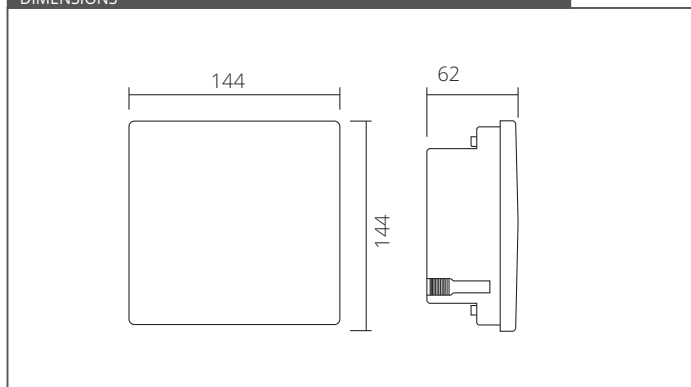
DIMENSIONS
