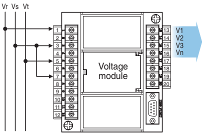
3P3W wiring
